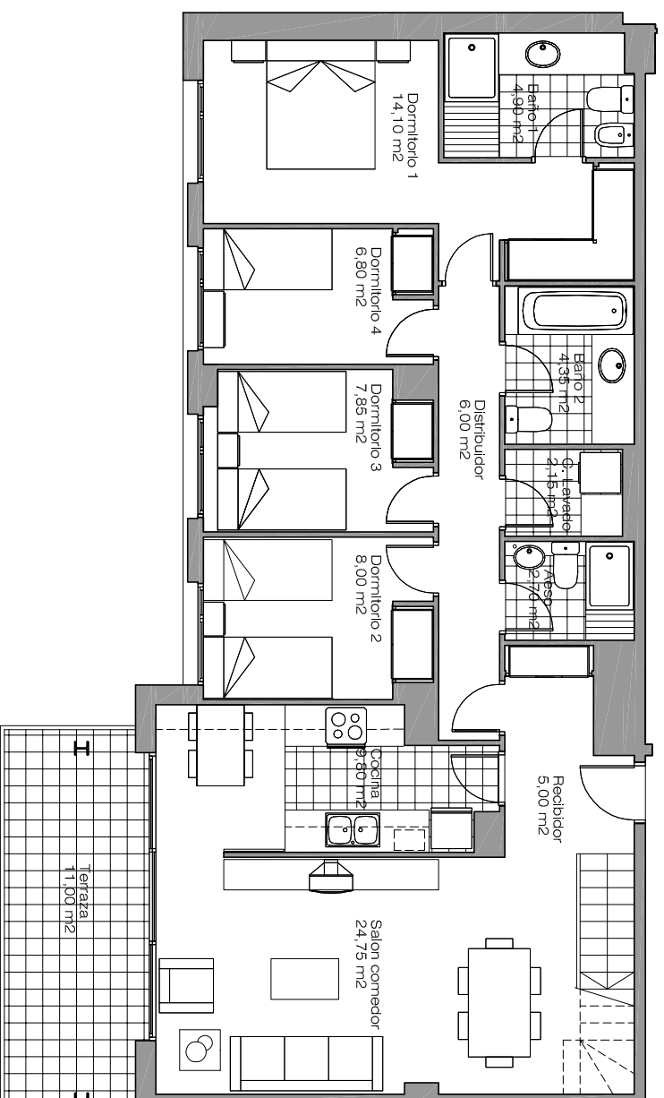
PLANTA TERCERA
